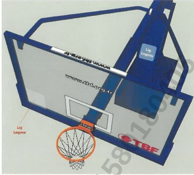
Çizim 1 - Arkalık işaretleri
