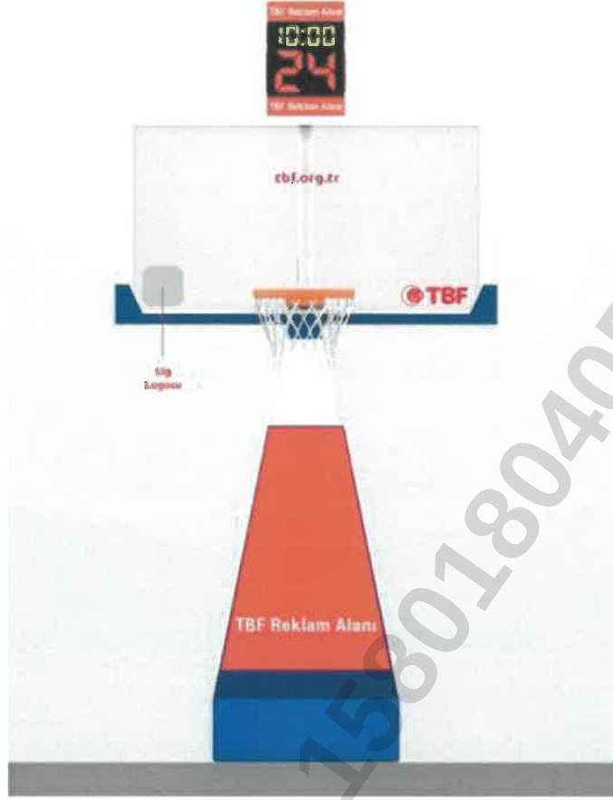
Çizim 4 - Arkalık ünitesi (ön)
